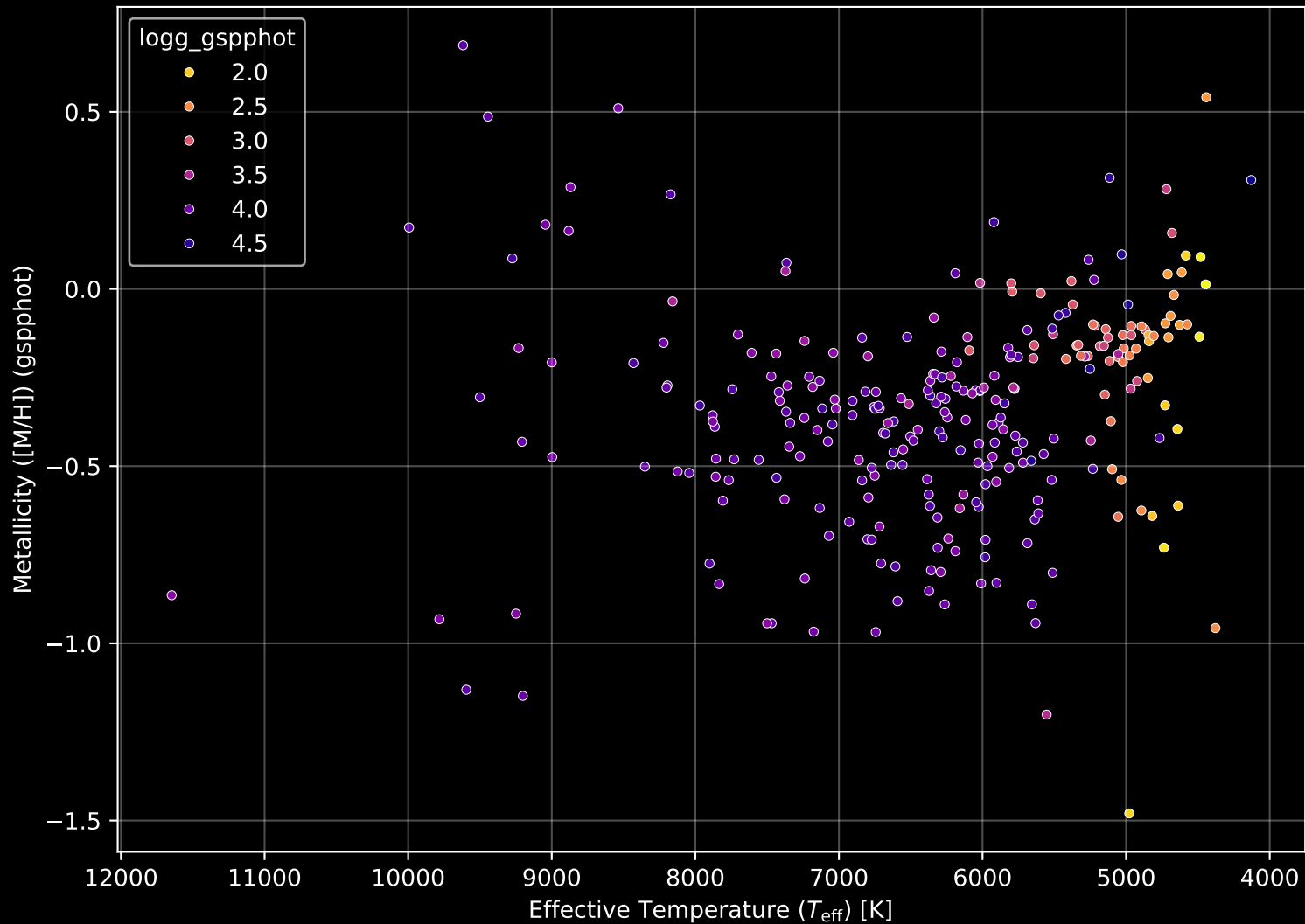
GALAH DR4 Field: [9218] Stellar Population Parameters (n= 279)
