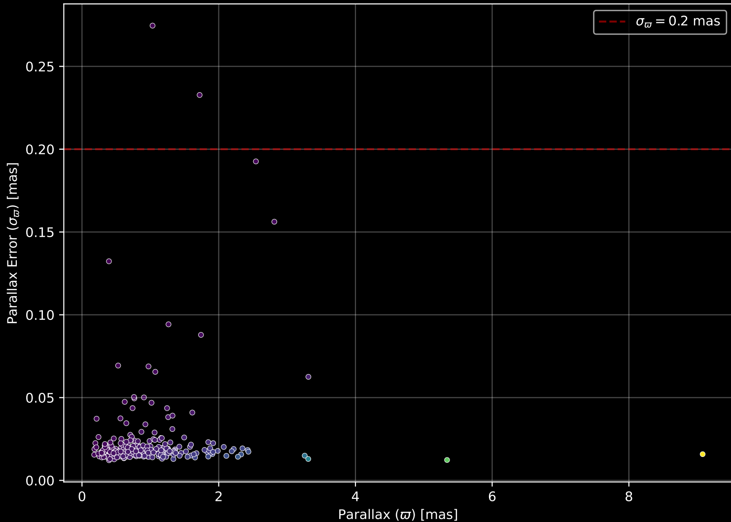
GALAH DR4 Field: [9218] Parallax Quality (n= 279)
