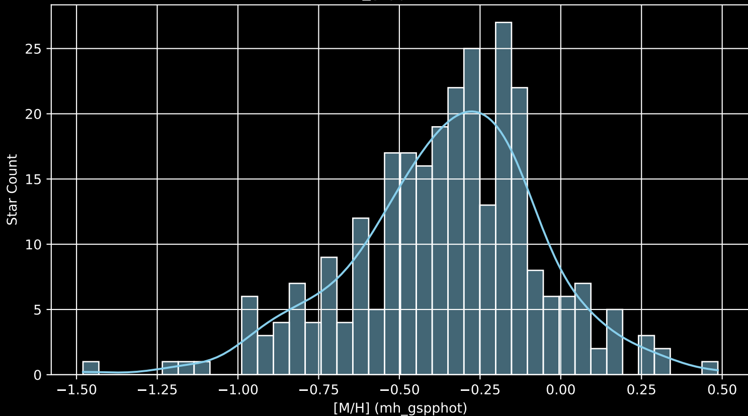
GALAH DR4 Field: [9218] [M/H] (mh_gspphot) (n= 276)
