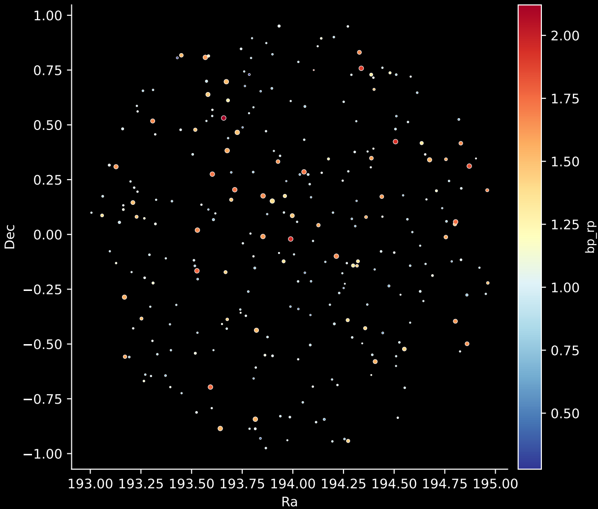
GALAH DR4 Field: [9218] Stars: 279
